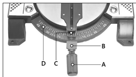
Рисунок 7. Модель BELMASH MS B-305
