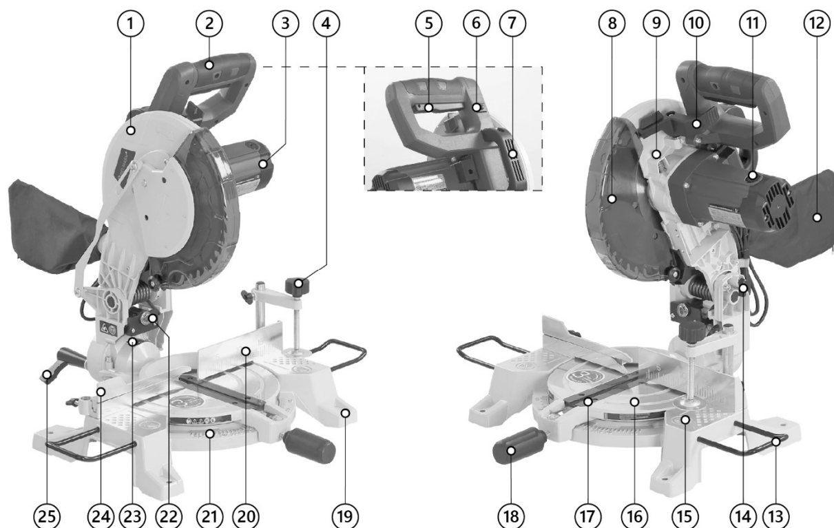
Рисунок 1 Основные элементы BELMASH MS B-255
